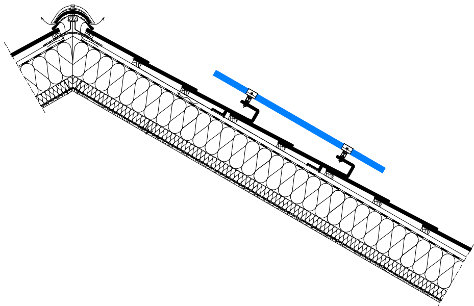
PRZEKRÓJ B-B
